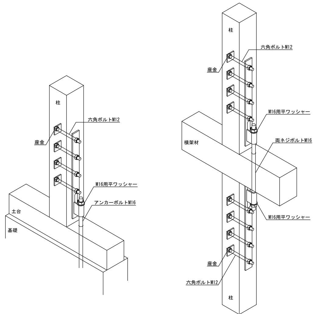
ホールダウンU 20kN用
