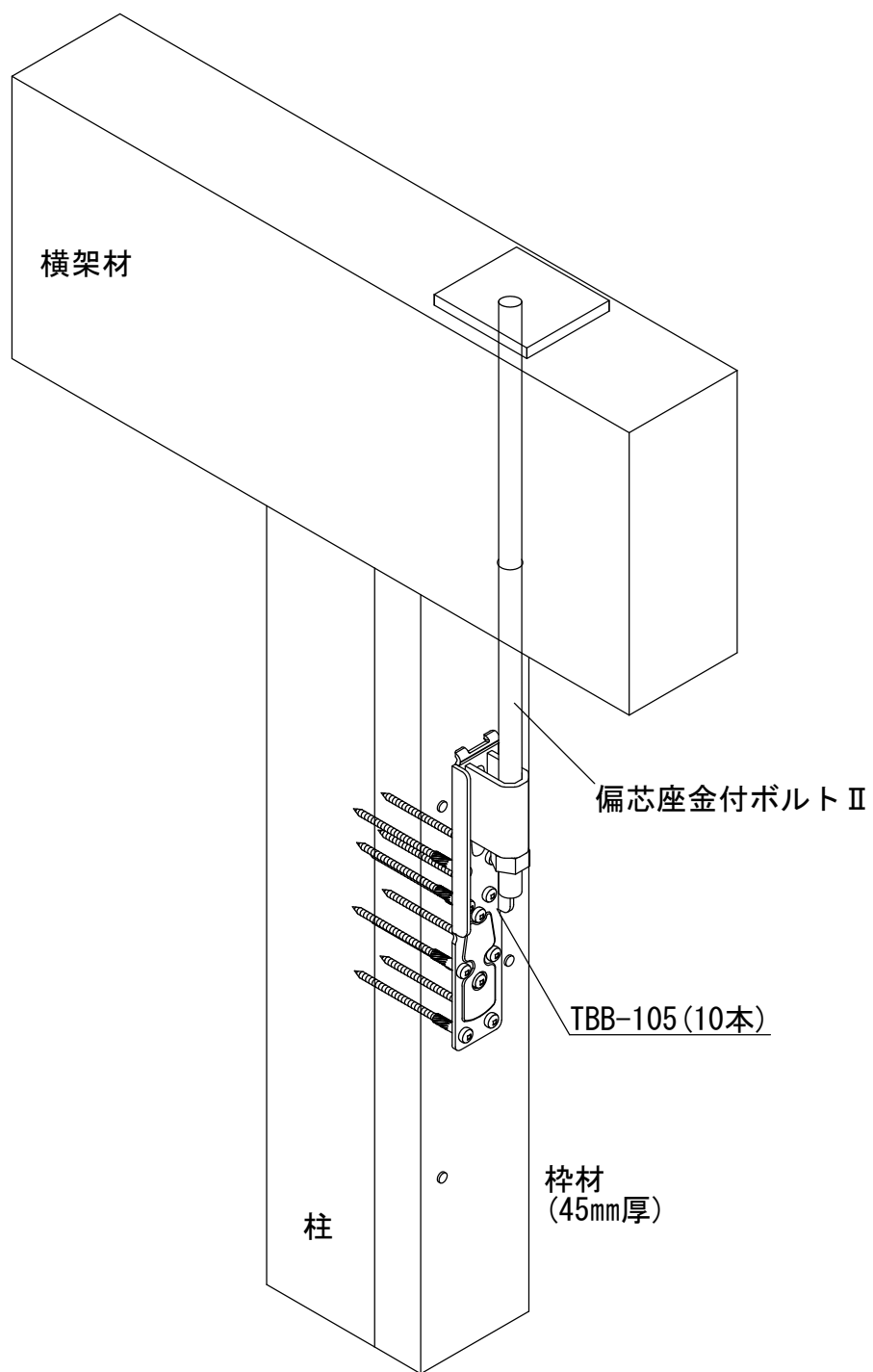
枠材用ビスどめホールダウンHi-L
