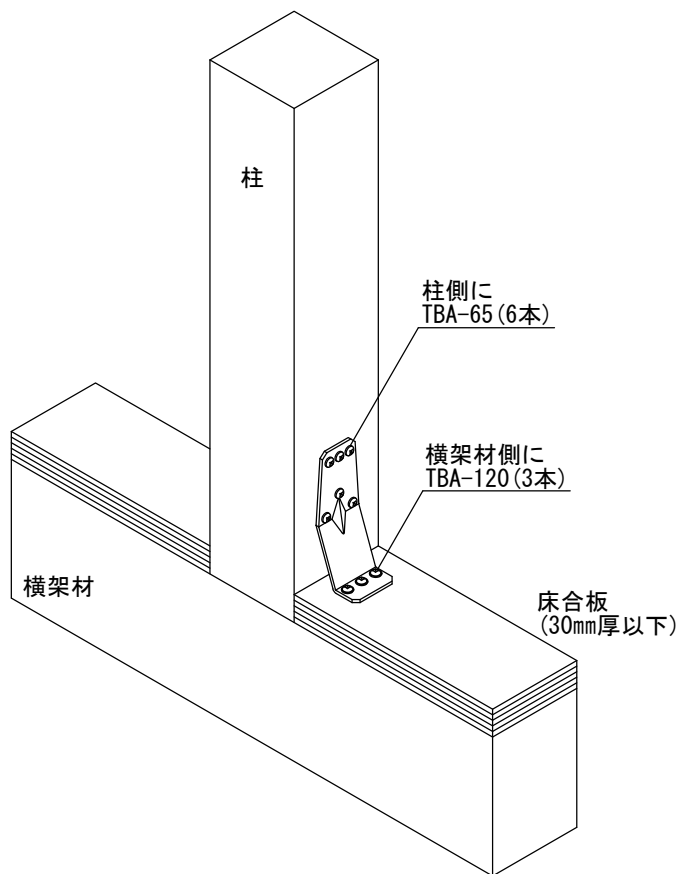
オメガコーナー15kNⅡ床合板仕様
