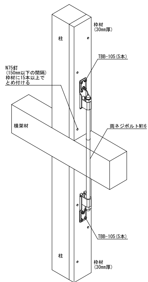
桟材用ビスどめホールダウンHi-M
