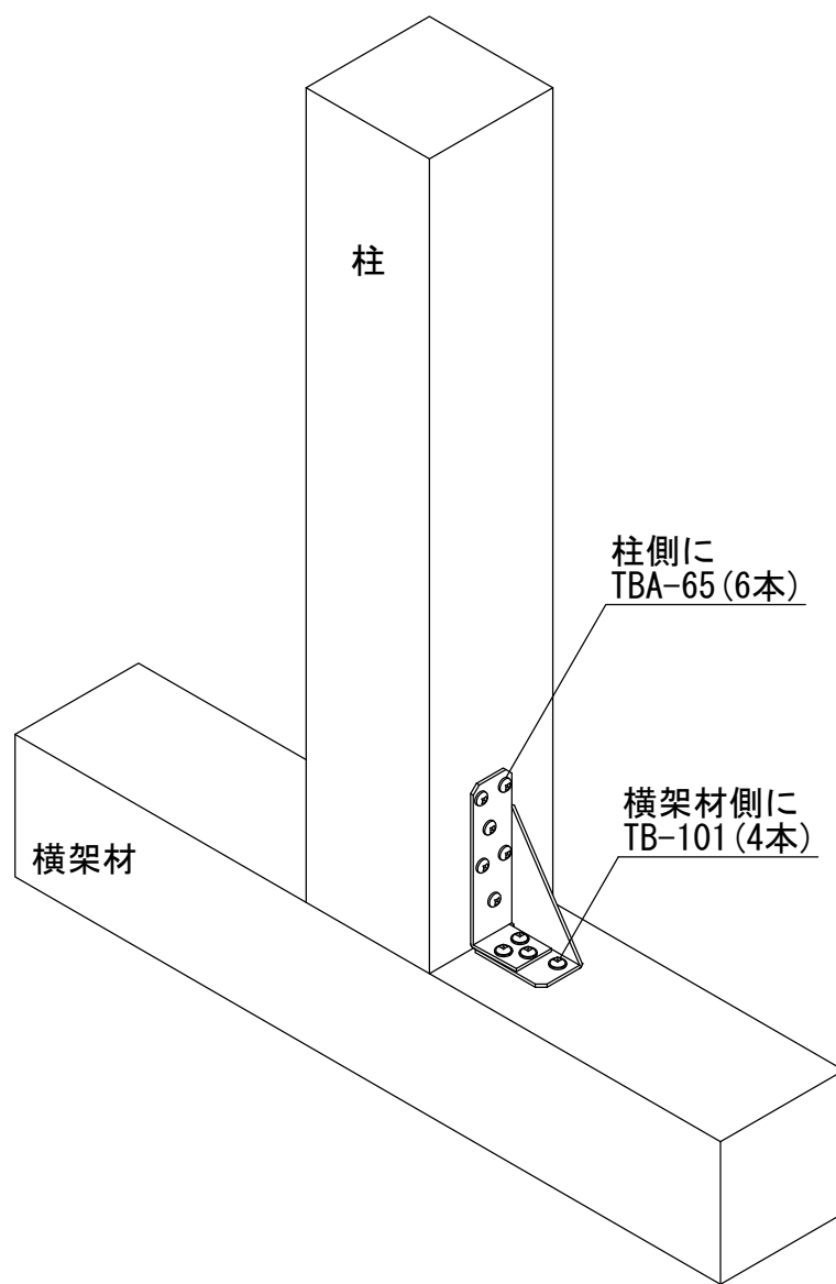
ホールダウンコーナー10kN用
