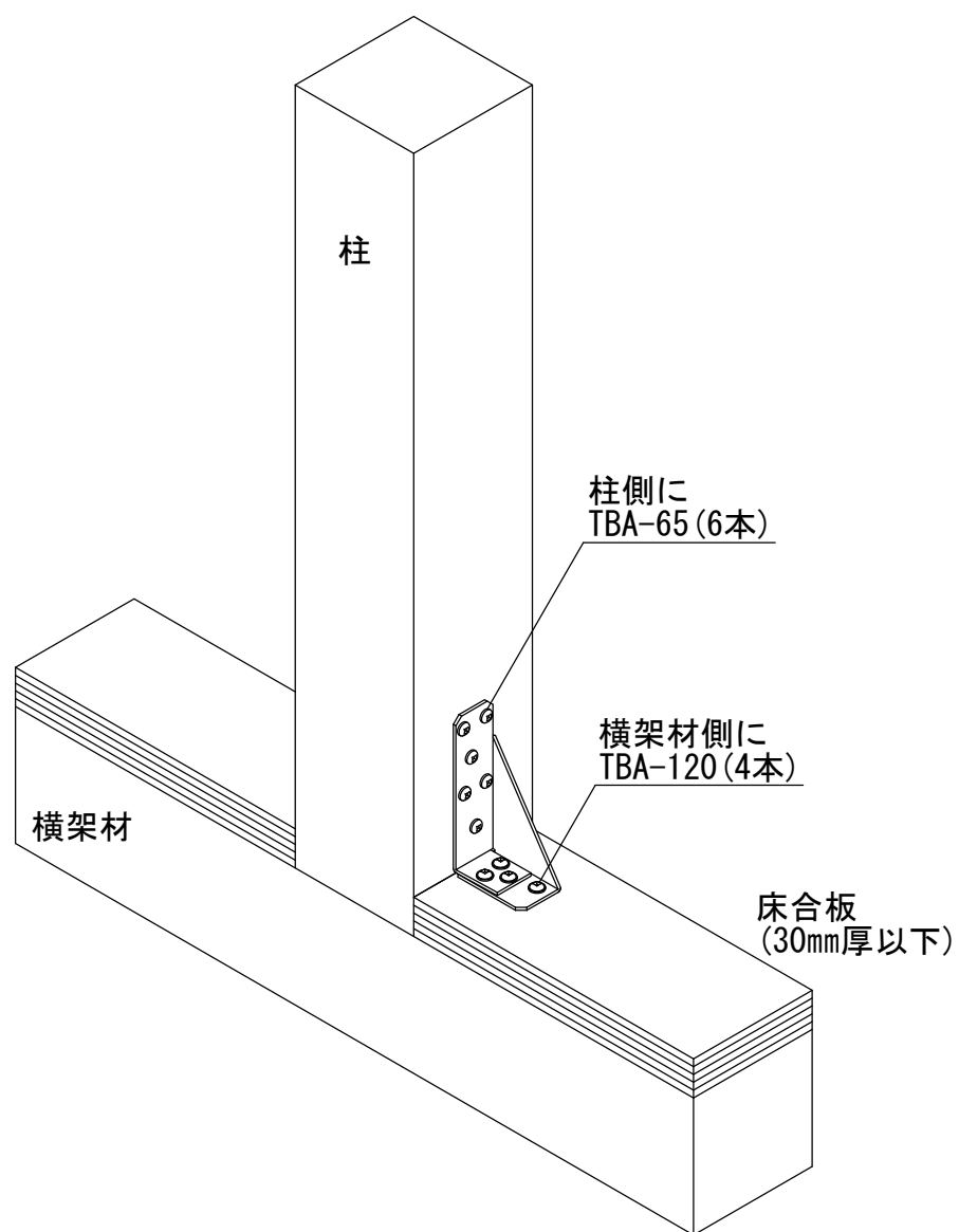
ホールダウンコーナー床合板仕様Ⅱ
