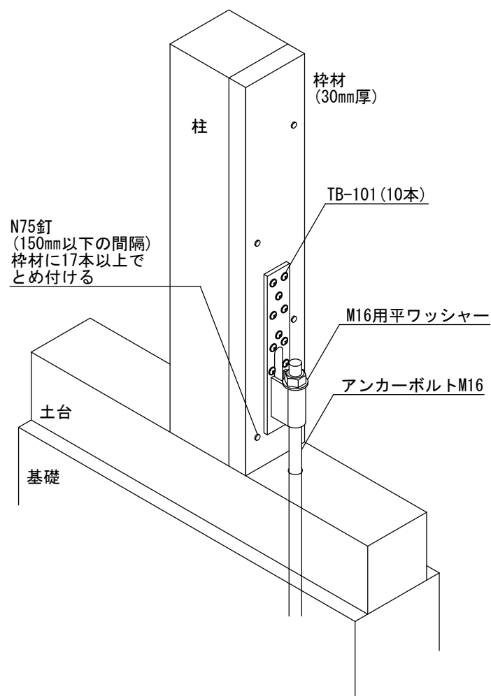
柱材用ビスどめホールダウンU 25kN用
