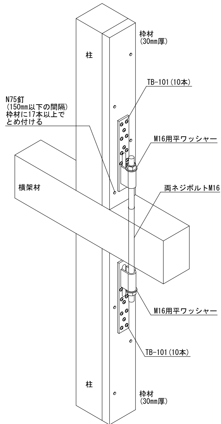
柱材用ビスどめホールダウンU 25kN用
