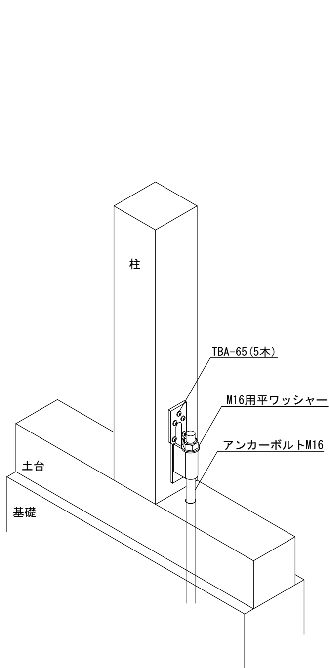
ビスどめホールダウンU 15kN用
