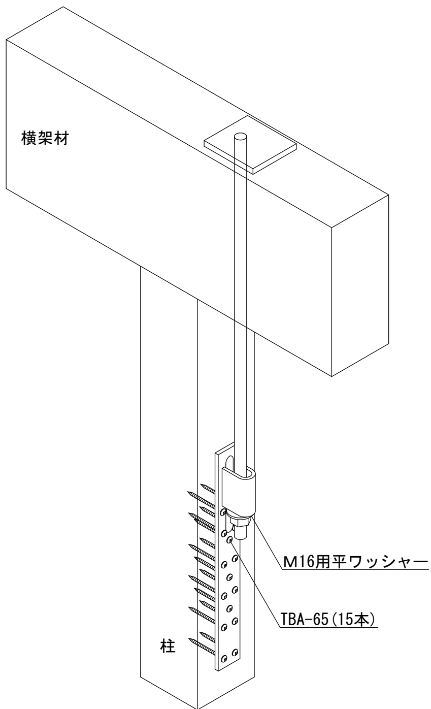
ビスどめホルダーU35kN用
