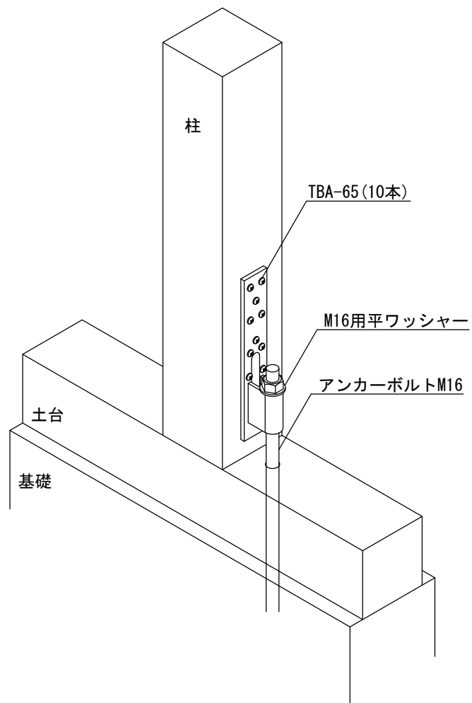
ビスどめホールダウンU 25kN用
