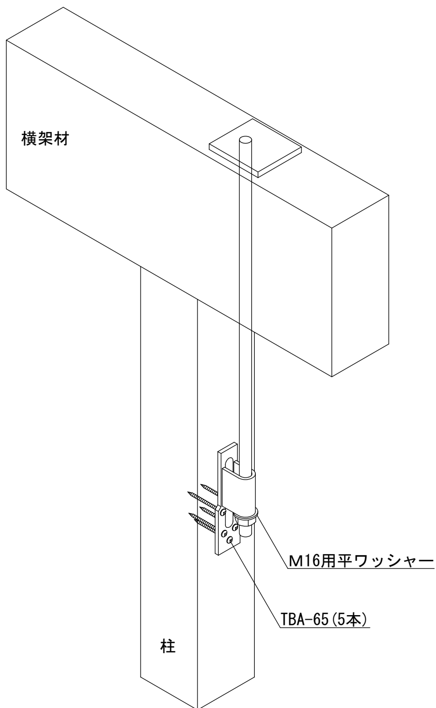
ビスどめホールダウンU15kN用
