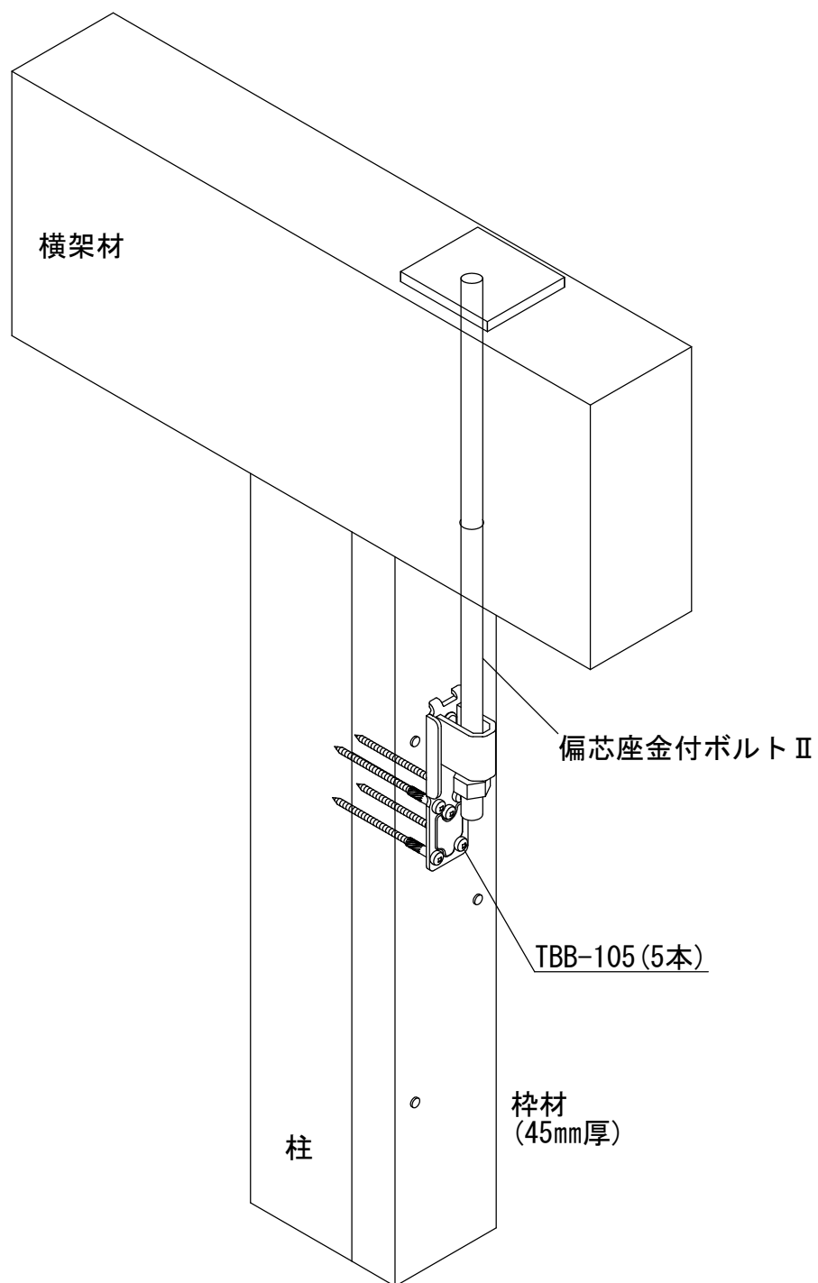
枋材用ビスどめホールダウンHi-M
