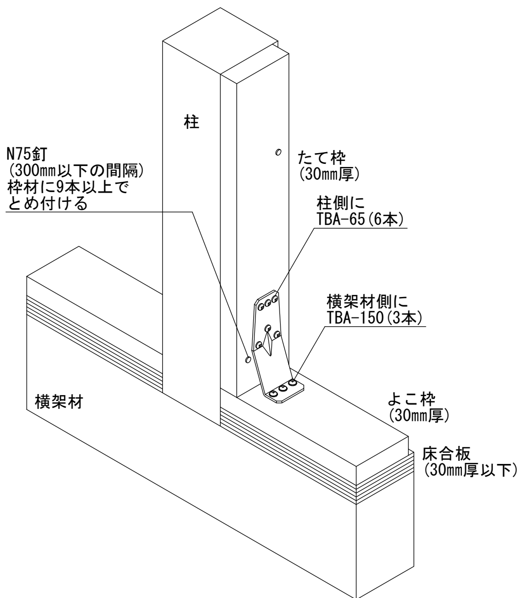
オメガコーナー15kNⅡ床枠仕様
