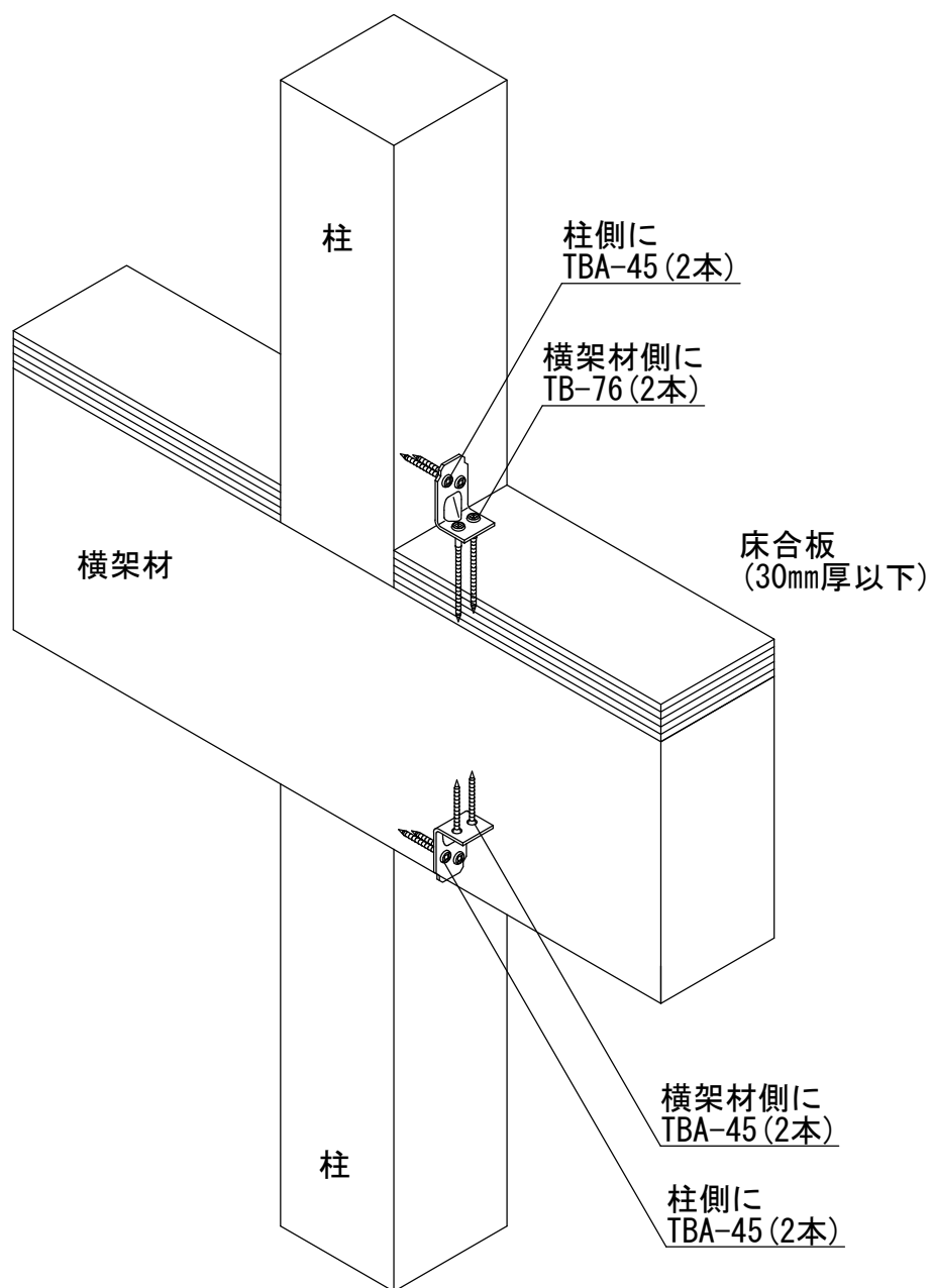
スモールコーナーⅡ 床合板仕様
