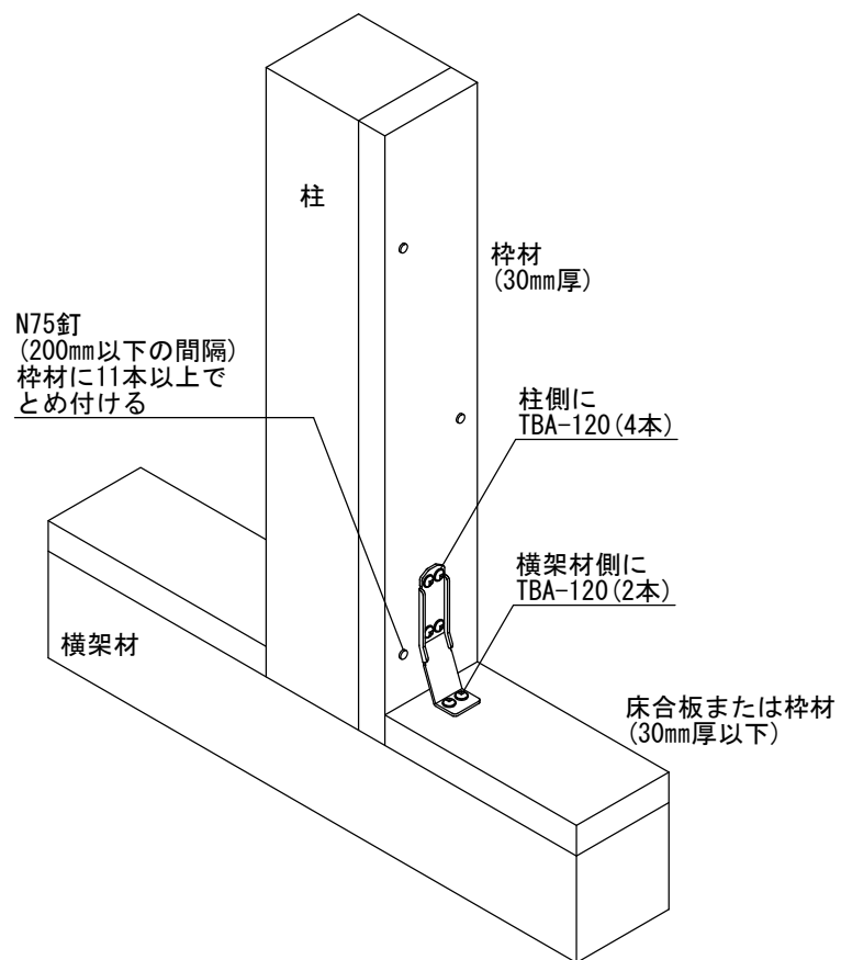
シナーコーナー枠材仕様
