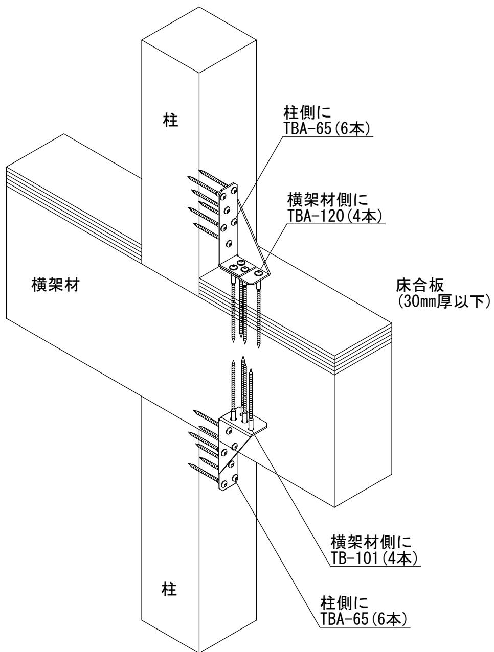
ホールダウンコーナー床合板仕様Ⅱ
