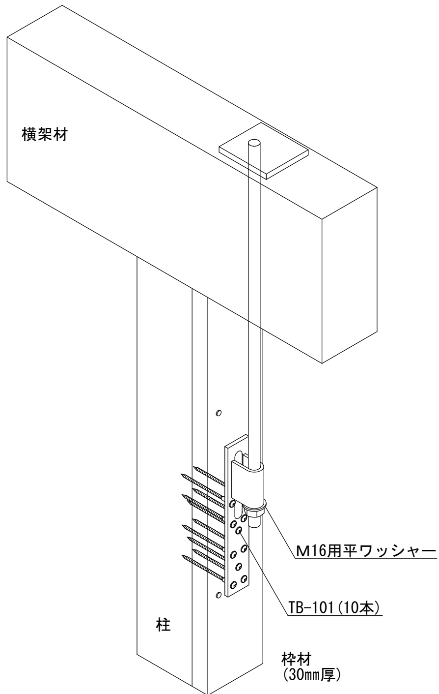
栓材用ビスどめホールダウンU25kN用
