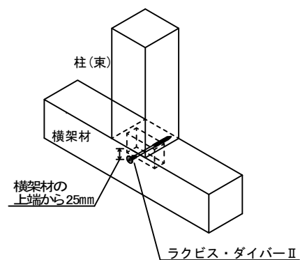
【ほぞ打ち】
