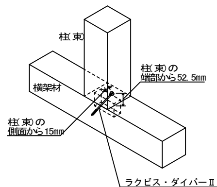
【斜め打ち】
