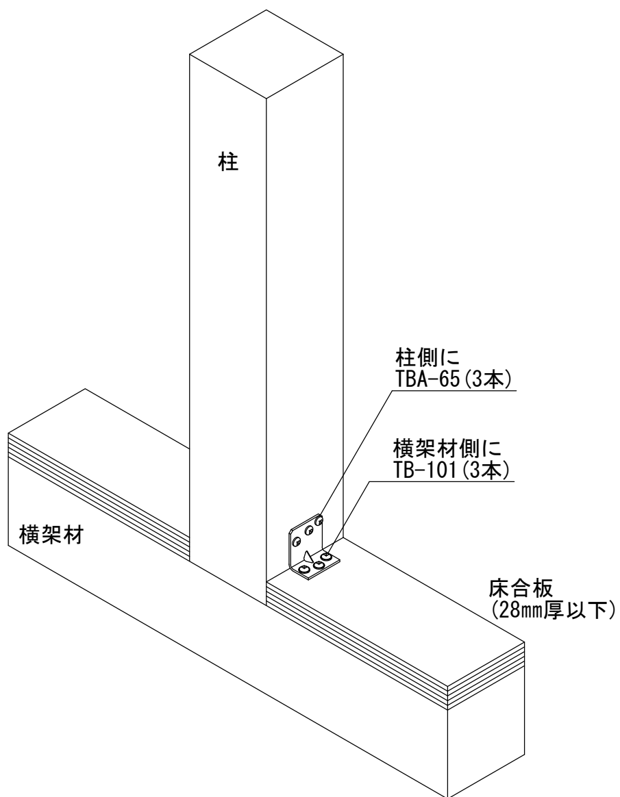
リトルコーナー床合板仕様
