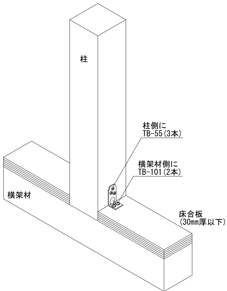
コンパクトコーナー床合板仕様
