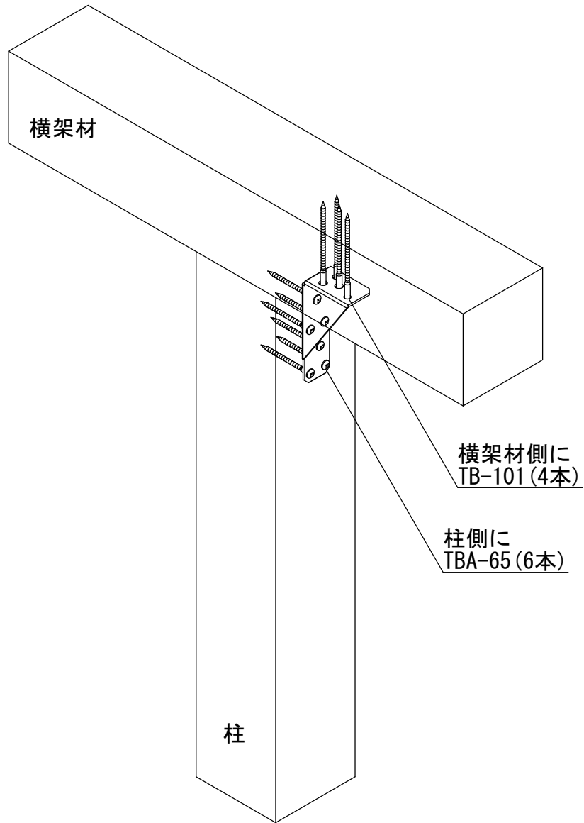
ホールダウンコーナー10kN用
