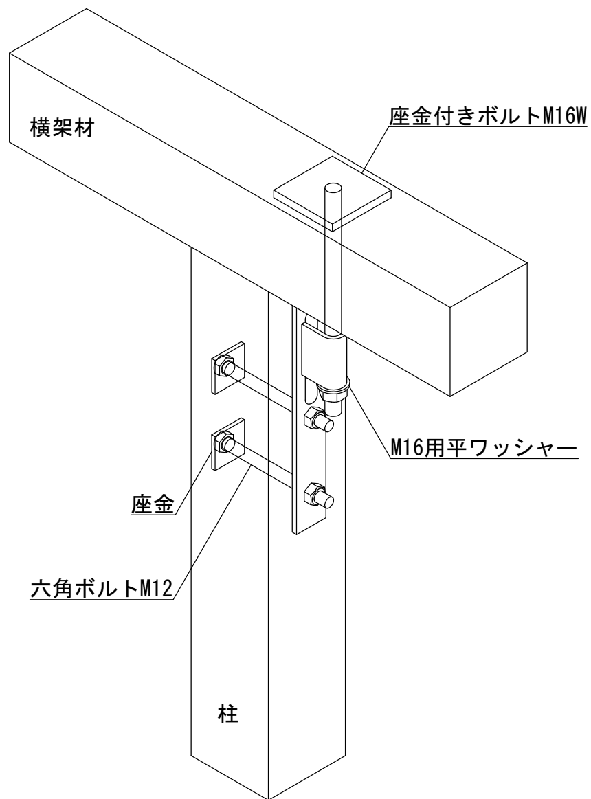
ホルダウンス U10kN用
