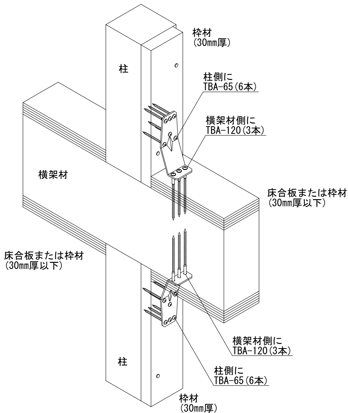
オメガコーナー15kNⅡ床合板仕様
