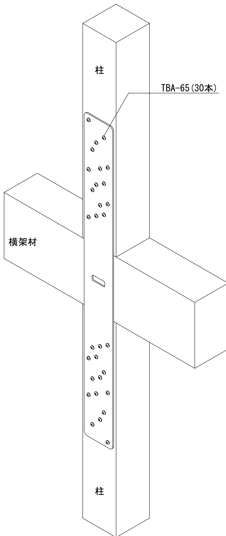
HDジョイント 39kN用ロングタイプ
