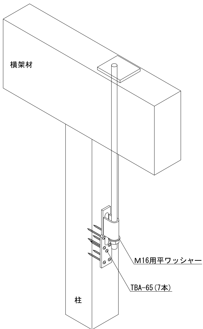
ビスどめホルダーU20kN用
