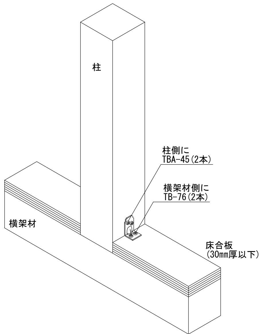
スモールコーナーⅡ床合板仕様
