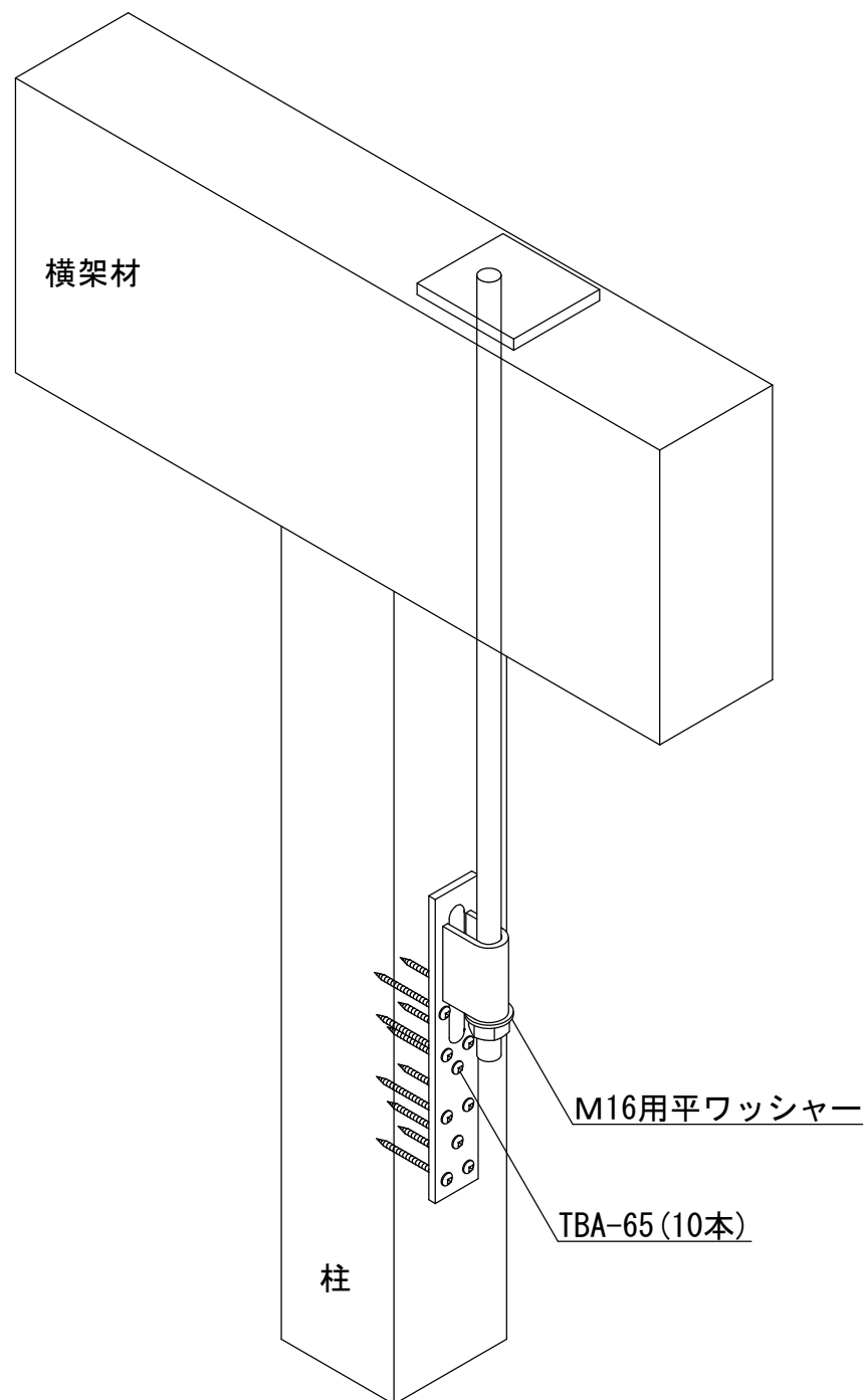
ビスどめホルダーU25kN用
