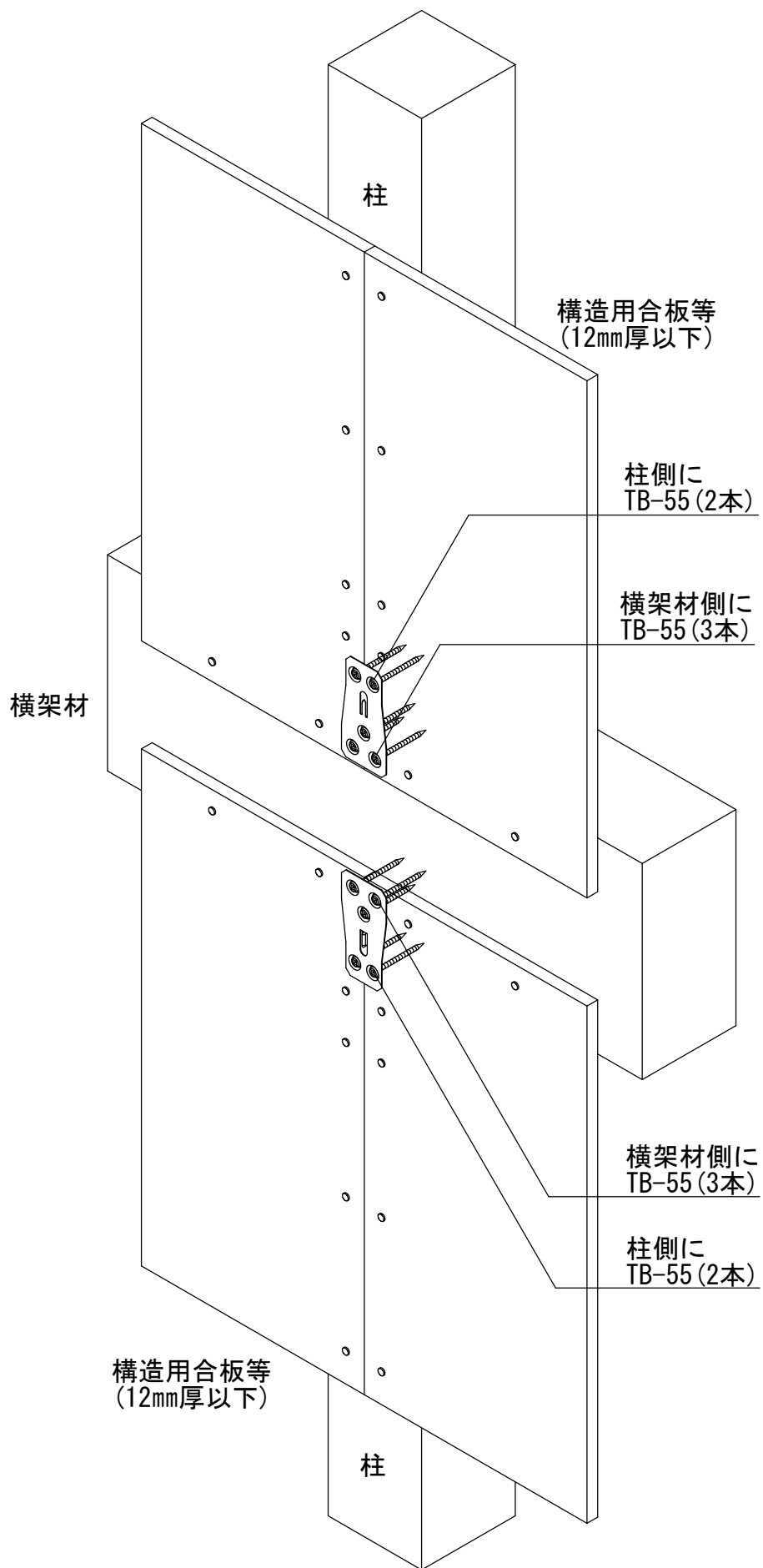
フラットプレートスリム合板仕様
