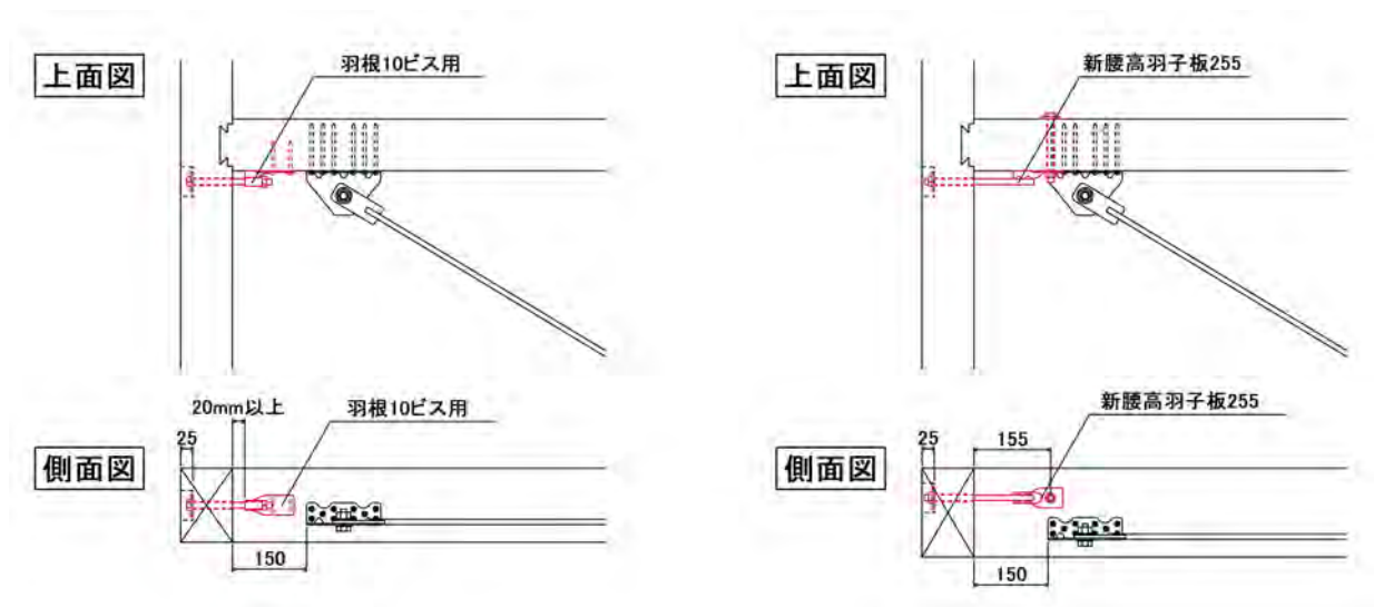
勾配用オメガメタルブレース端部金物と羽子板ボルトとの納まり確認図
