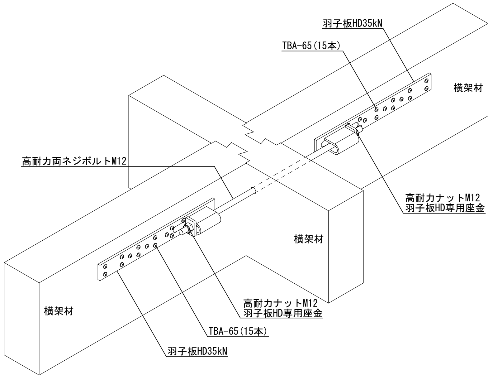
羽子板HD35kN <両引きセット>
