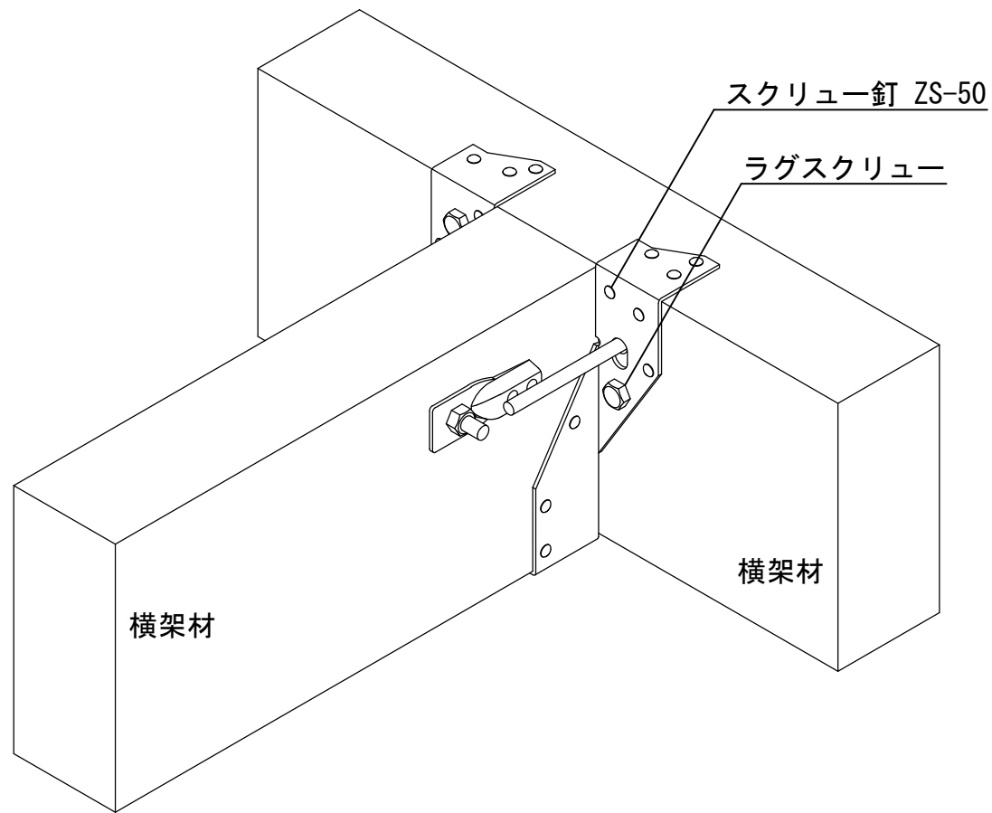
梁受け金物(ツメあり)
