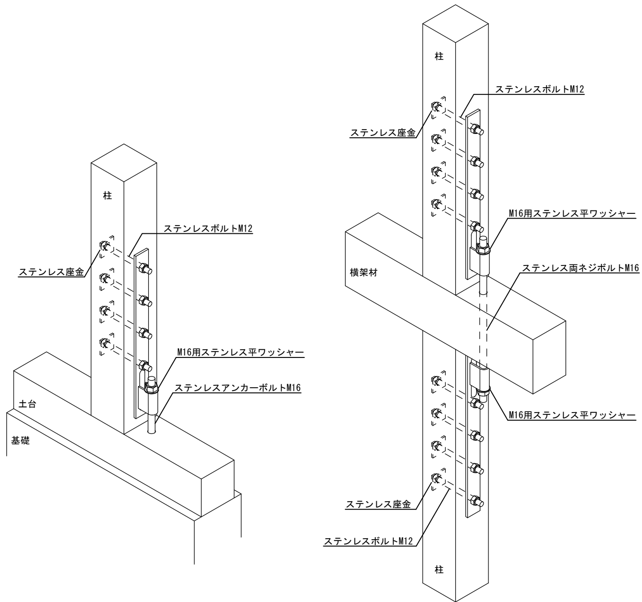
ステンレスホールダウンU 20kN用
