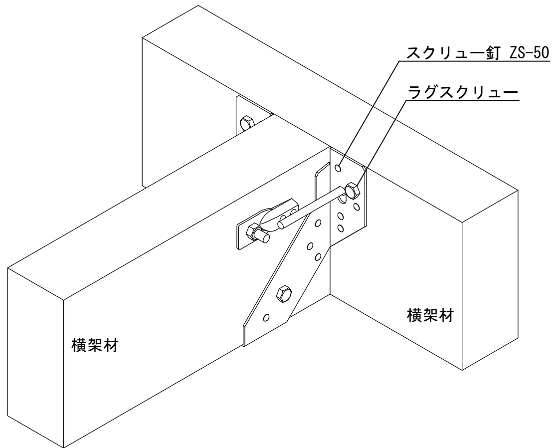
外付け梁受け金物
