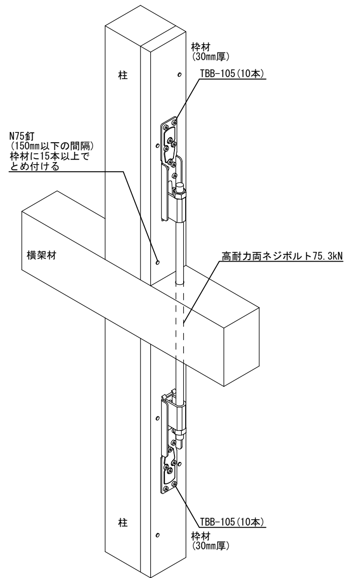
splice 材用ビスどめホルダウンHi-L
