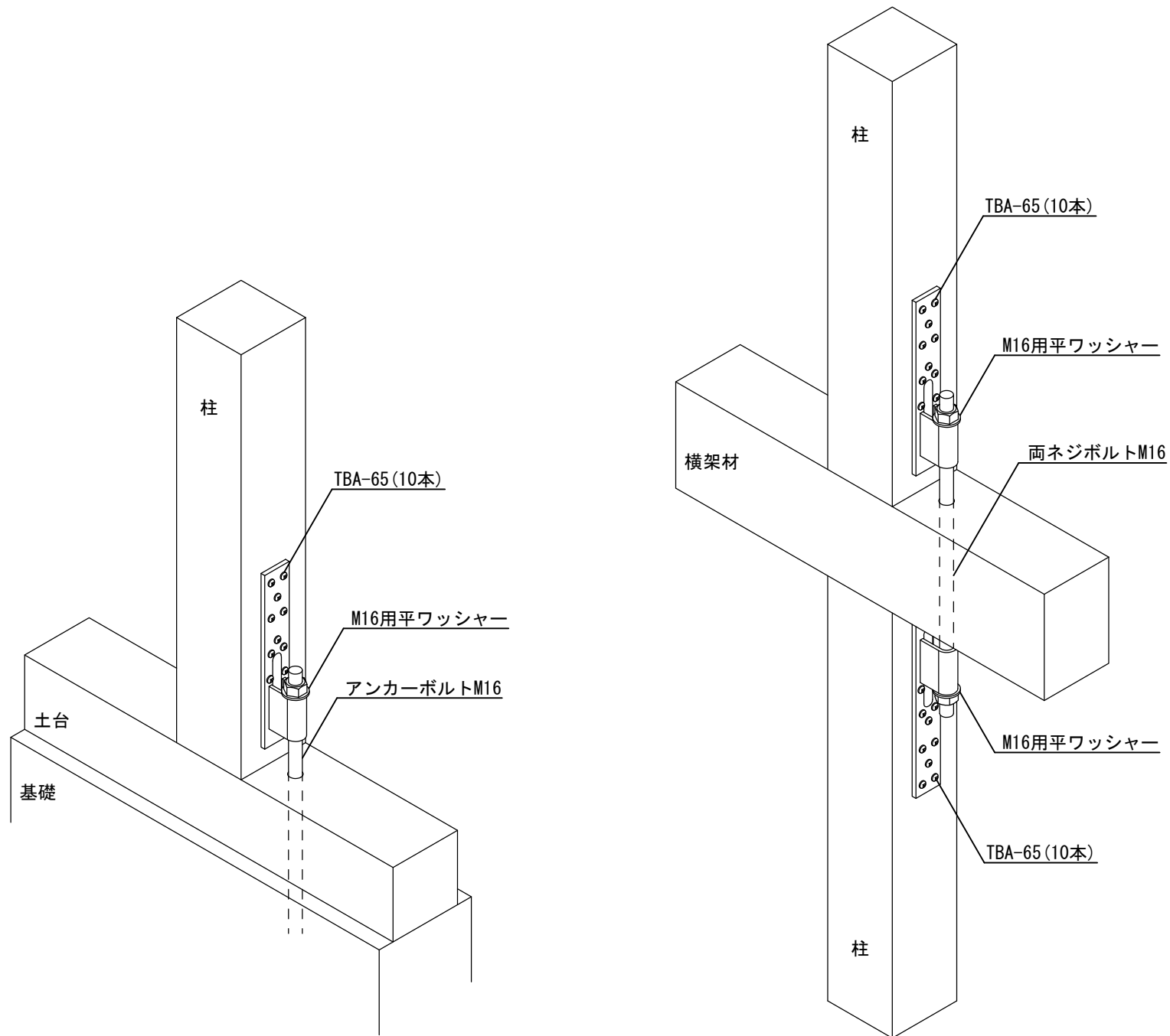
ビスどめホールダウンU 25kN用
