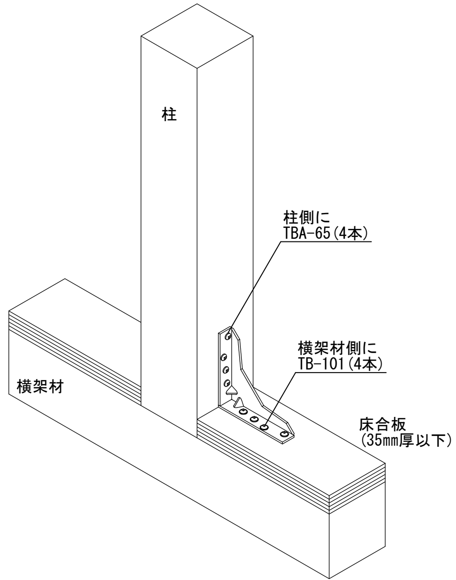
スリムプレート床合板仕様
