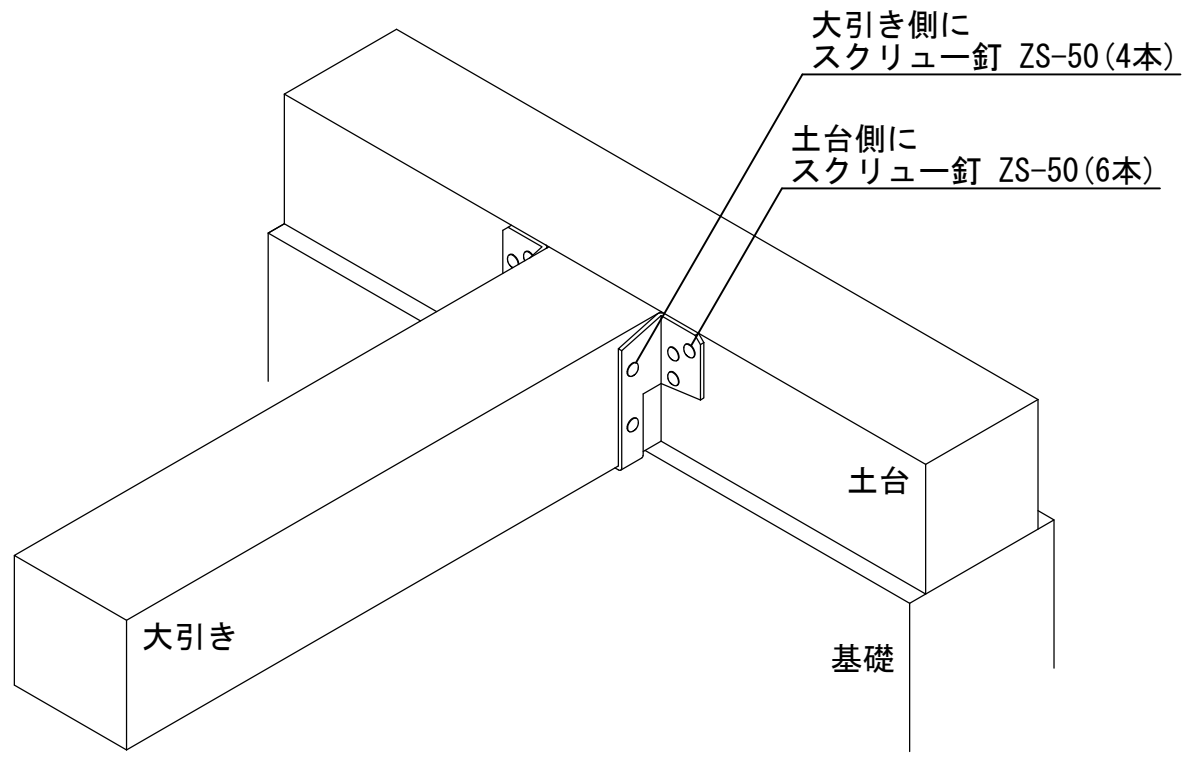
外折り大引き受け金物
