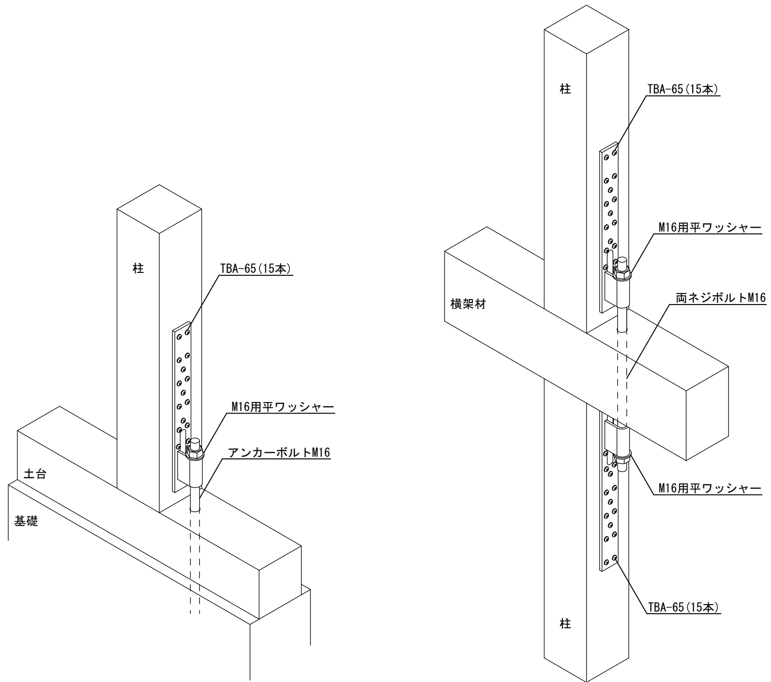
ビスどめホールダウンU 35kN用
