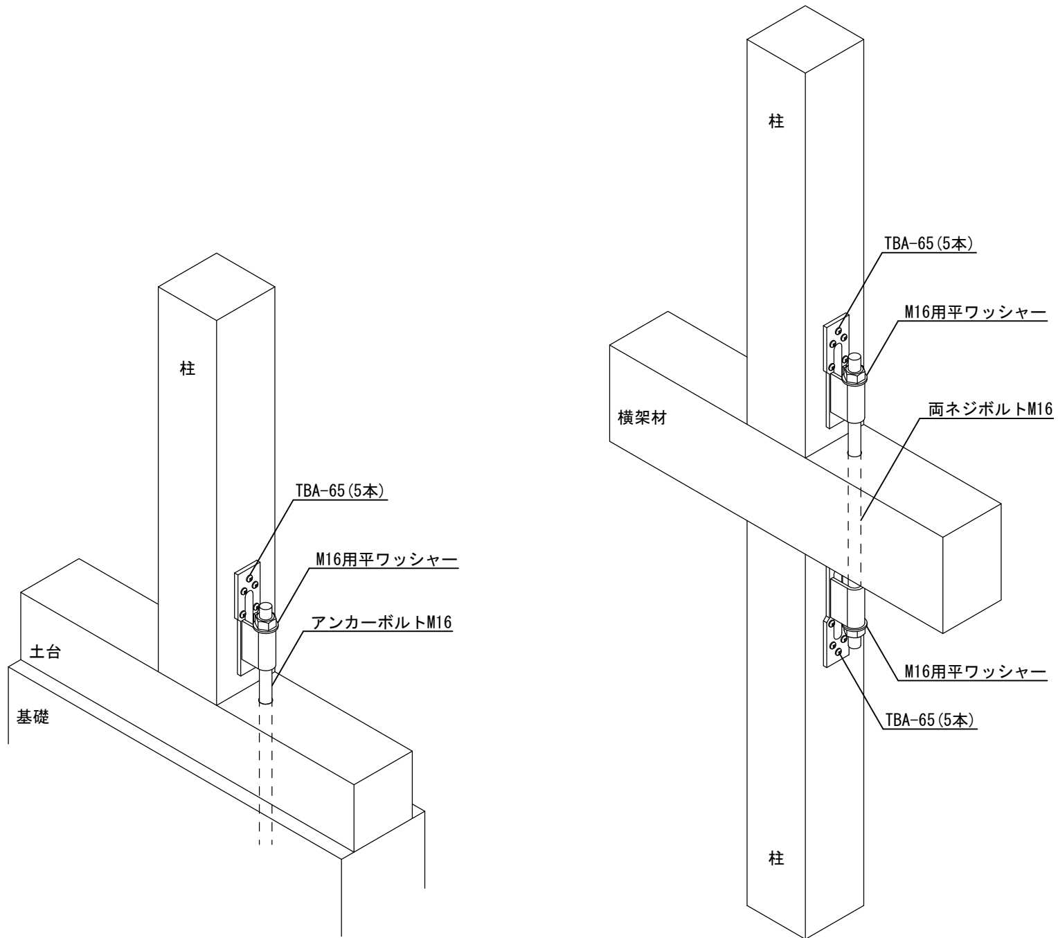
ビスどめホルダウN 15kN用
