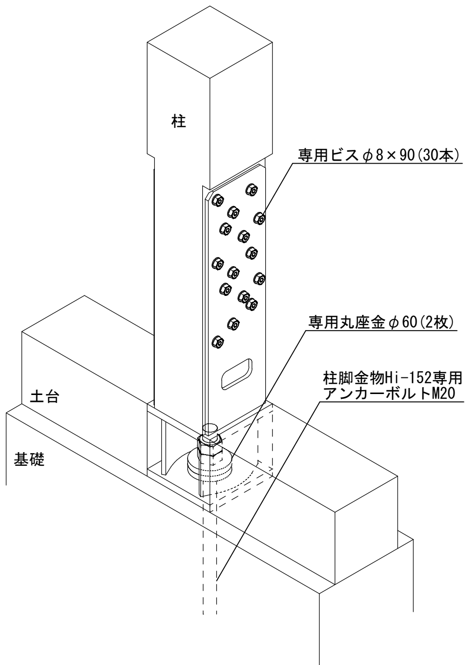
中大規模対応 柱脚金物Hi-152
