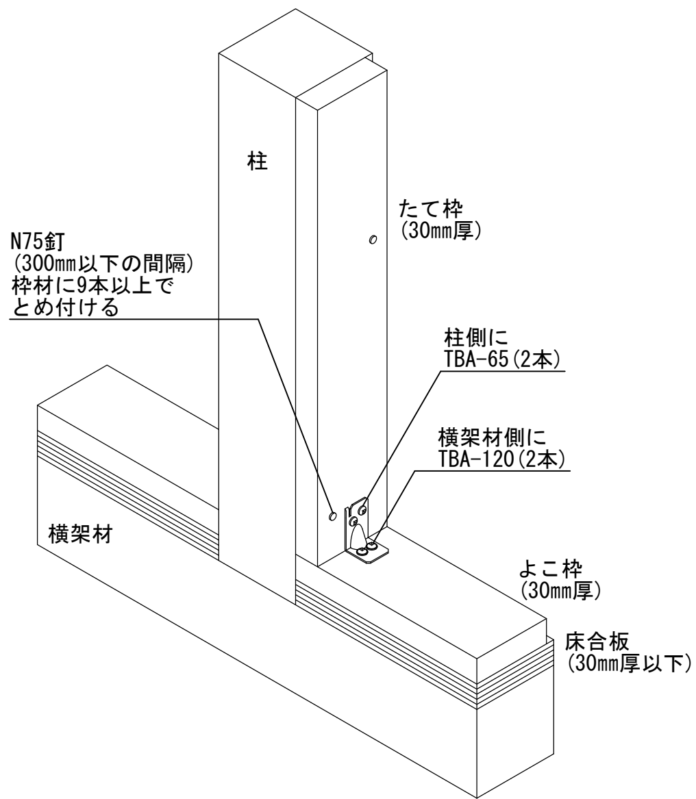
フックコーナー床枠仕様
