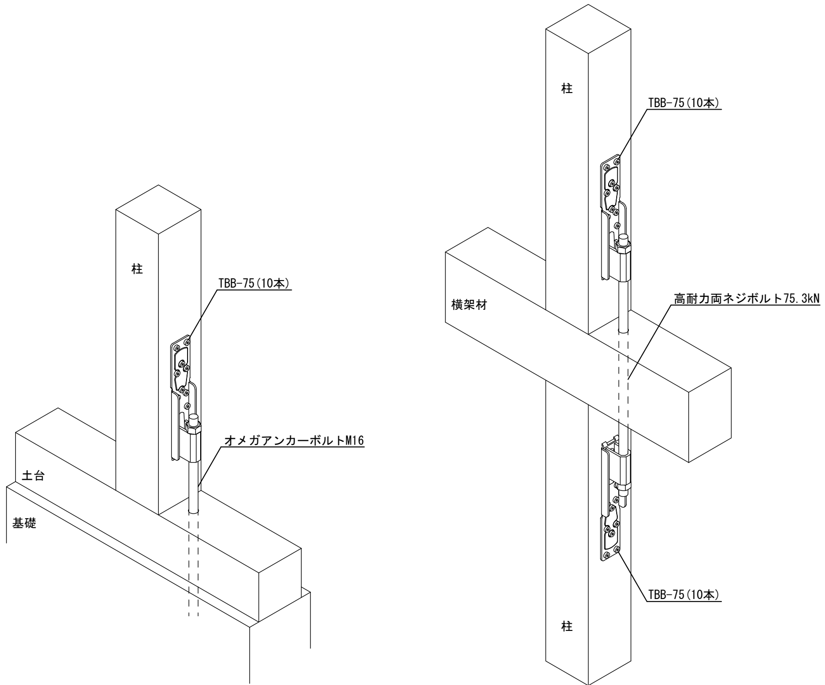
ビスどめホールダウンHi43
