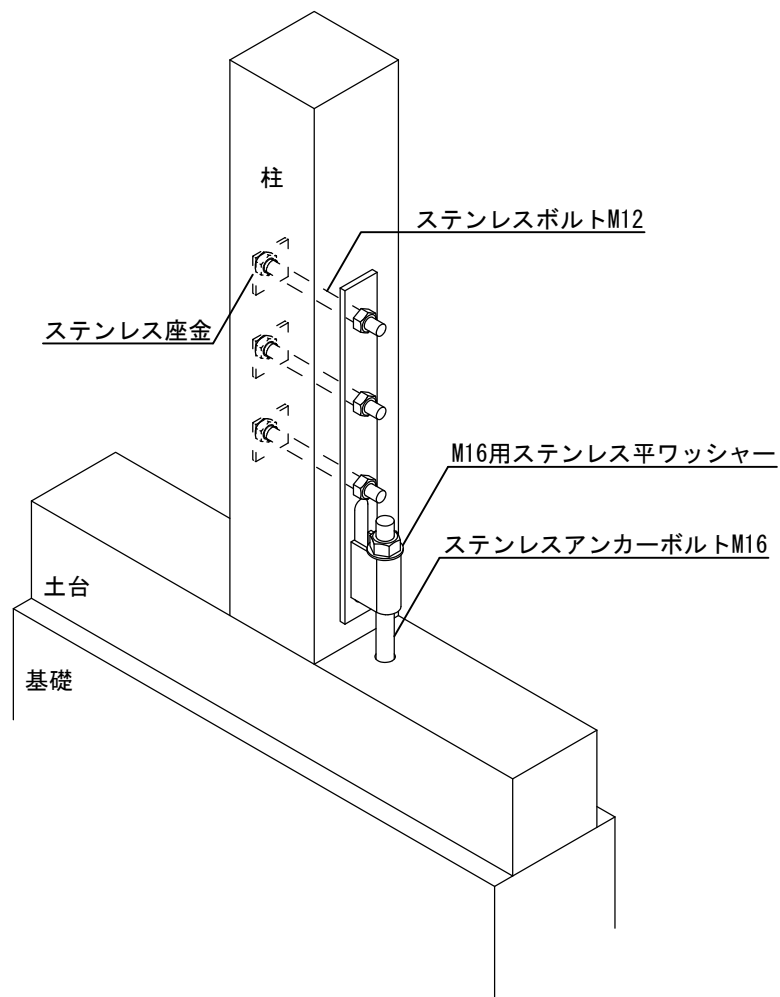
ステンレスホールダウンU 15kN用
