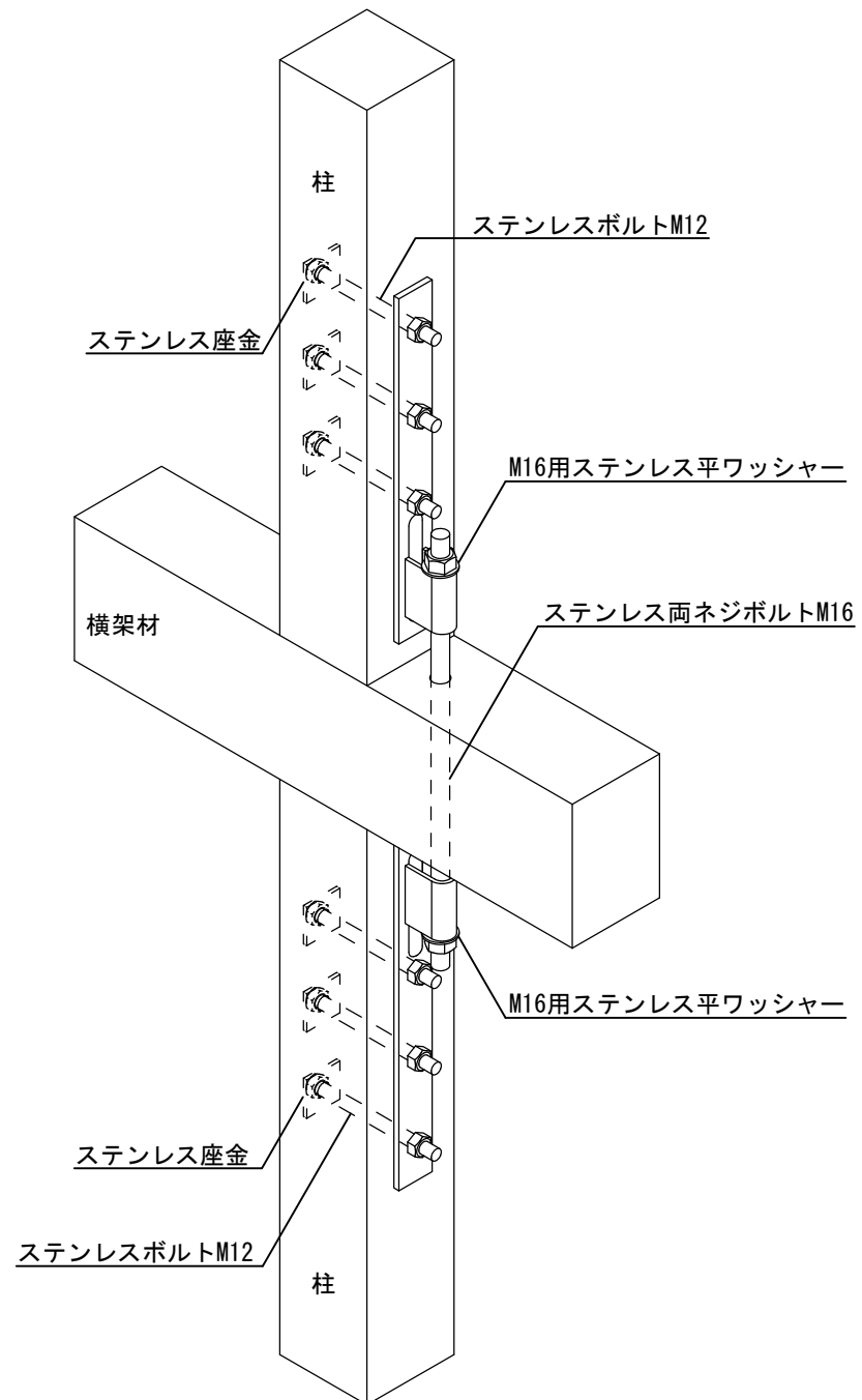
ステンレスホールダウンU 15kN用
