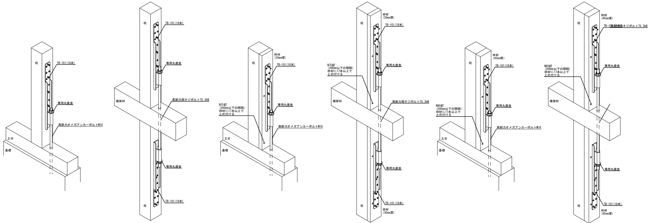
高耐力ホールダウンHi
