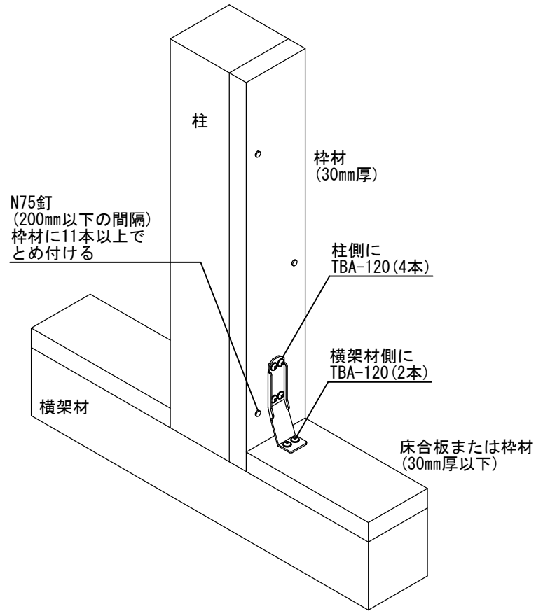
シナーコーナー柱材仕様
