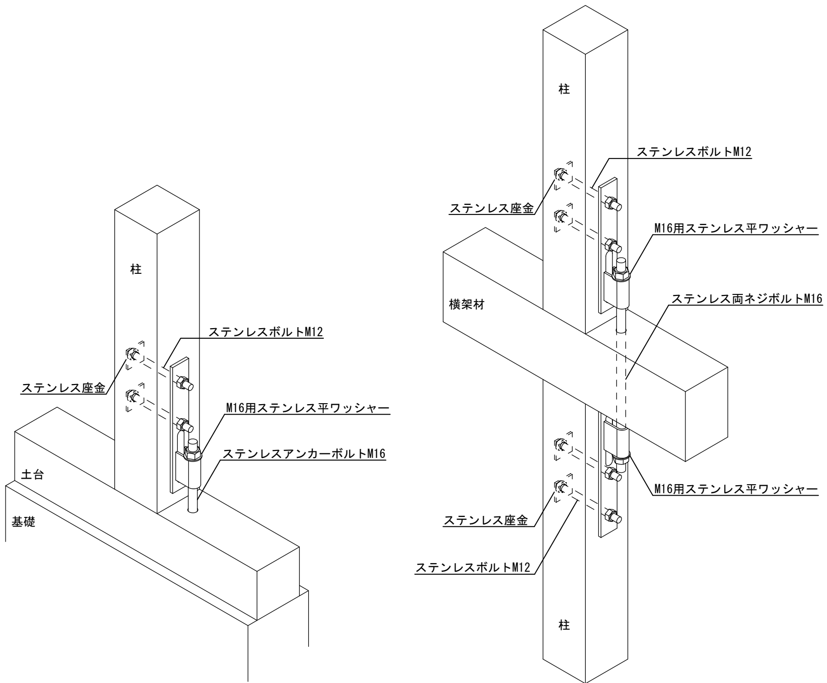
ステンレスホールダウンU 10kN用
