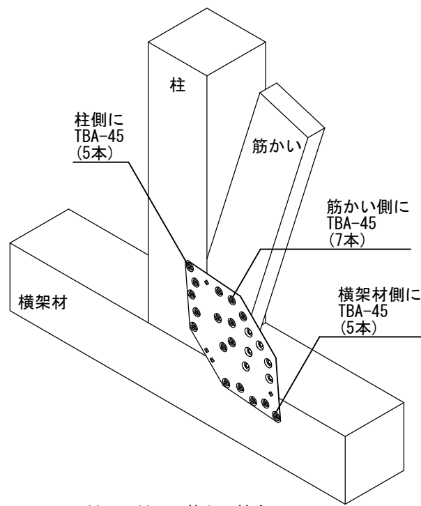
30mm × 90mmの筋かい接合
