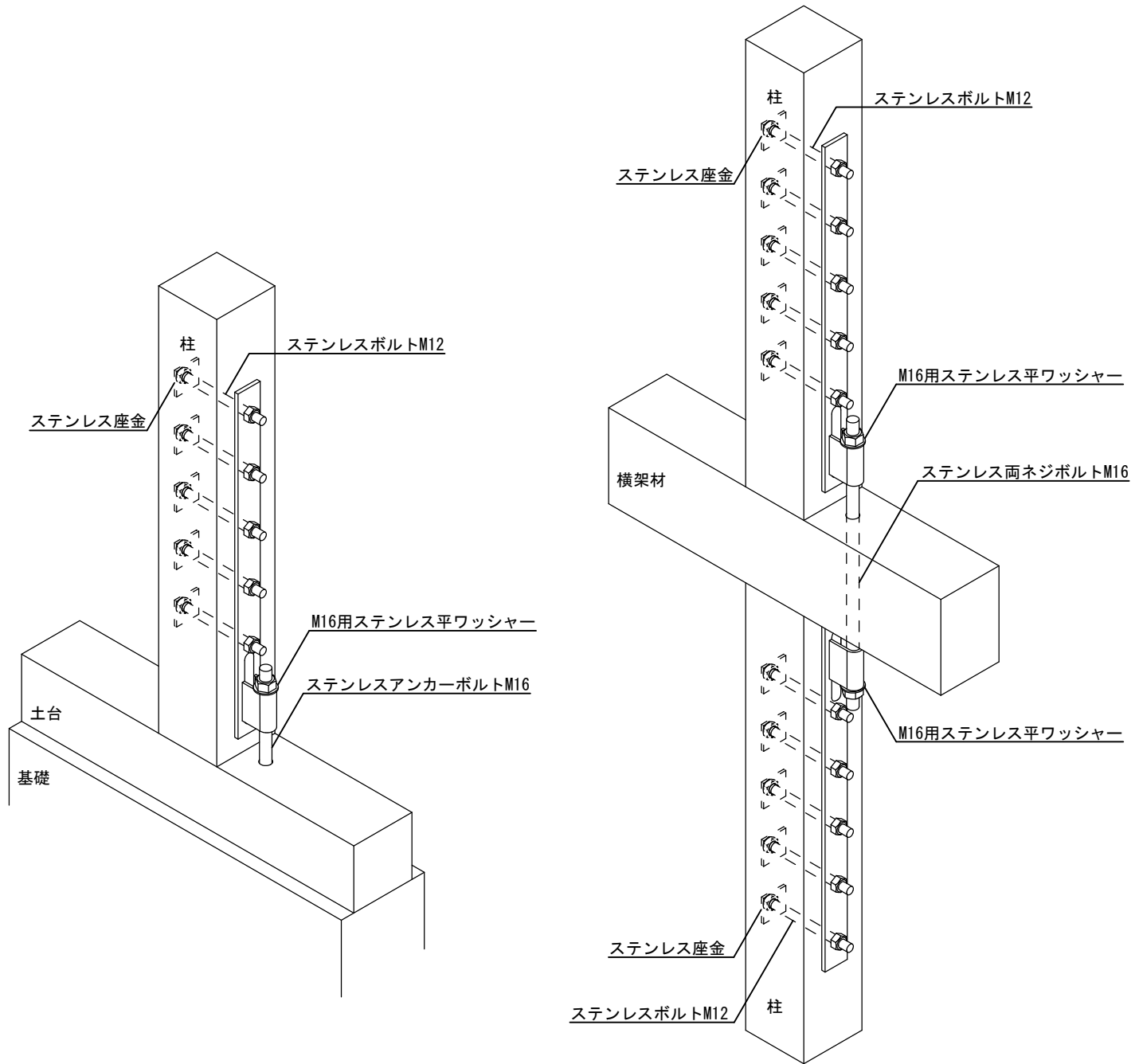
ステンレスホールダウンU 25kN用
