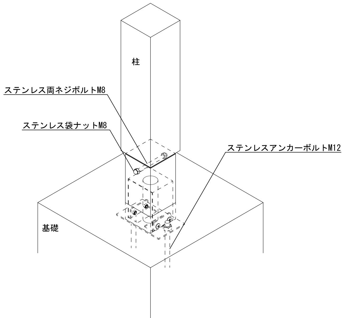
ステンレス装飾柱脚金物Sタイプ
